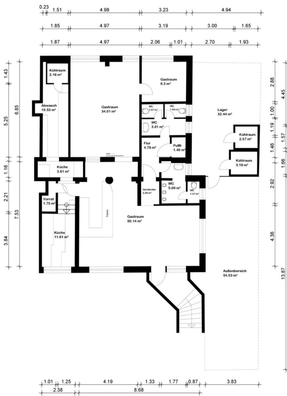
Grundriss
