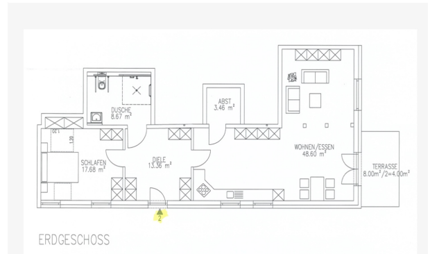
Grundriss_Whg2
