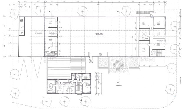
Obergeschoss
